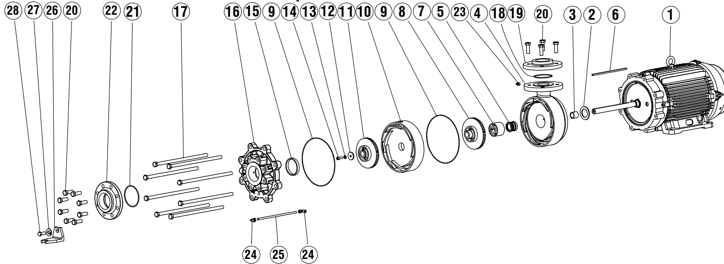
Vista Explodido Motobomba FMG IP55
