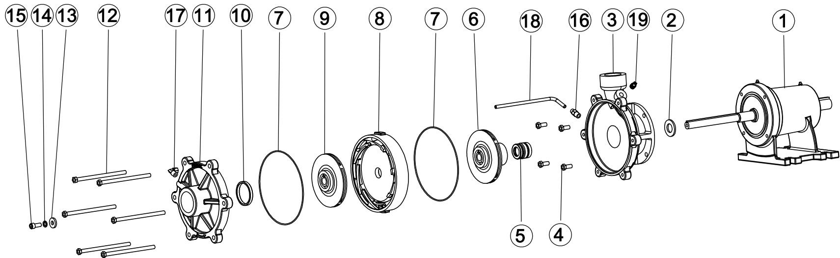
Vista explodida Mancalizada FMG
